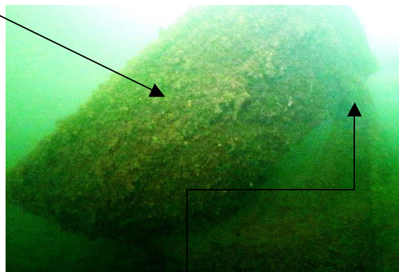
Ruderblatt geknickt
